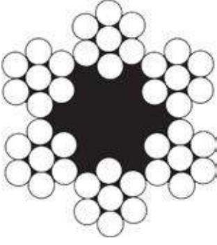
1x9 1(1+6+12) Kullanım Alanları Otomotiv Seracılık Kablo
